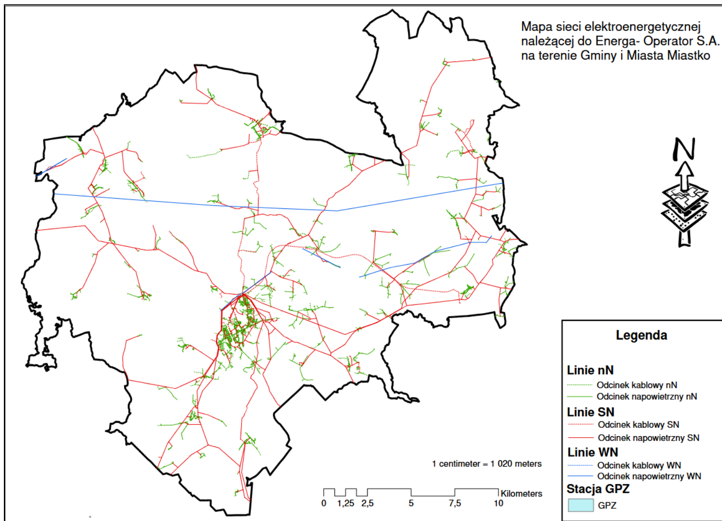
Rysunek 10. Przebieg sieci elektroenergetycznej na terenie gminy Miastko należącej do Energa-Operator SA
